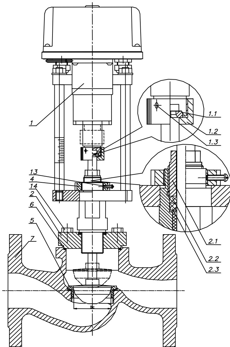
Рисунок 1. Общее устройство клапана КЗР 50/XX.Б-XX
