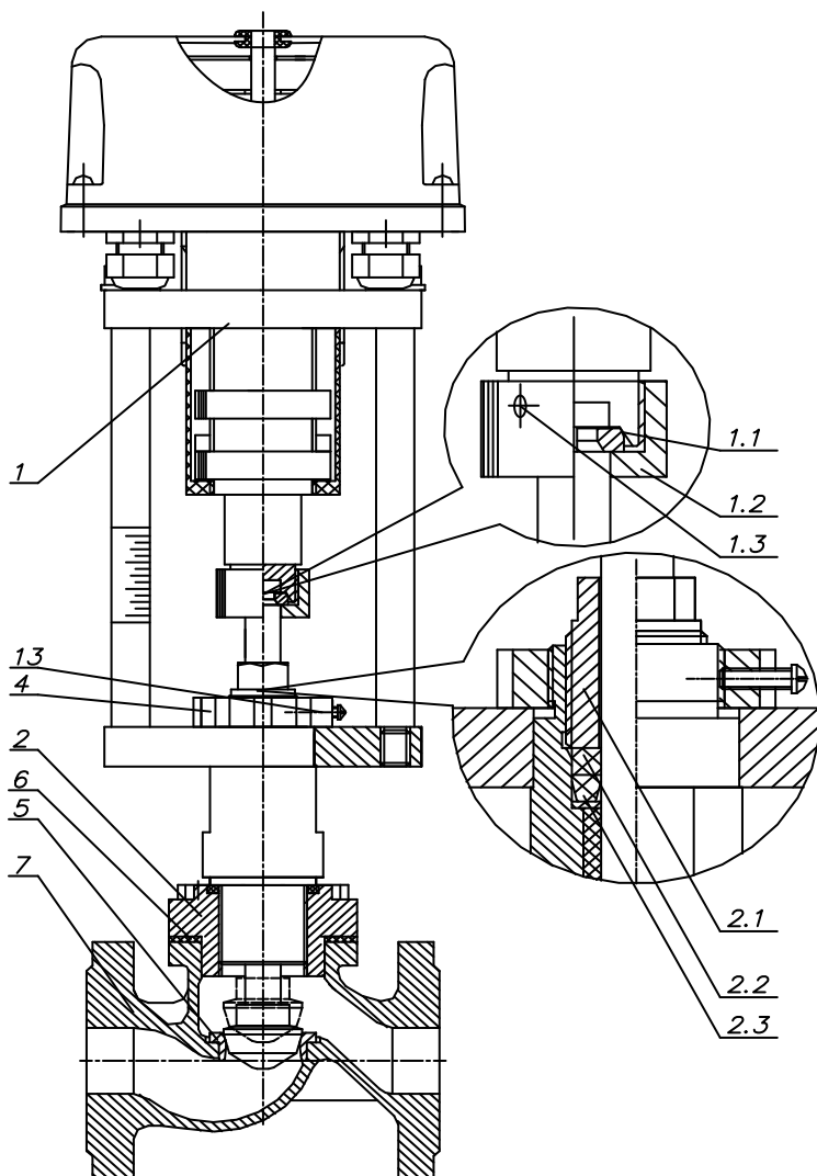
Рисунок 1. Общее устройство клапана КЗР-20/XX.Б-XX
