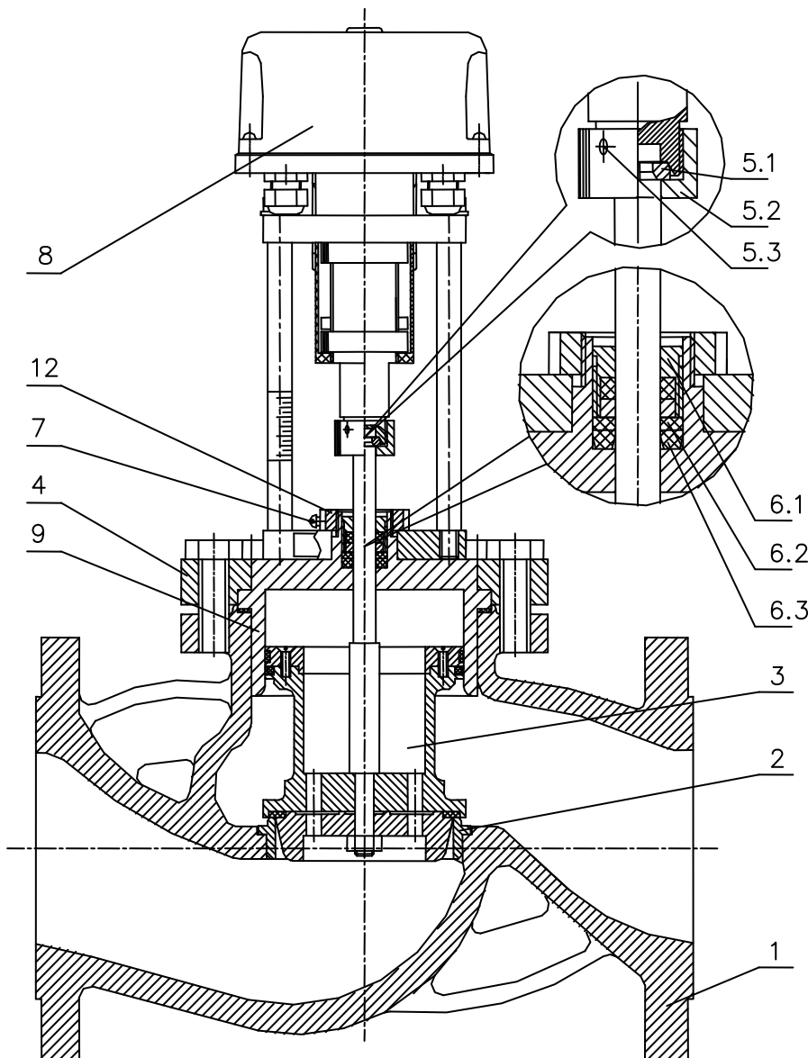
Рисунок 1 Общее устройство клапана КЗРр-150/145.Б-ХХ
