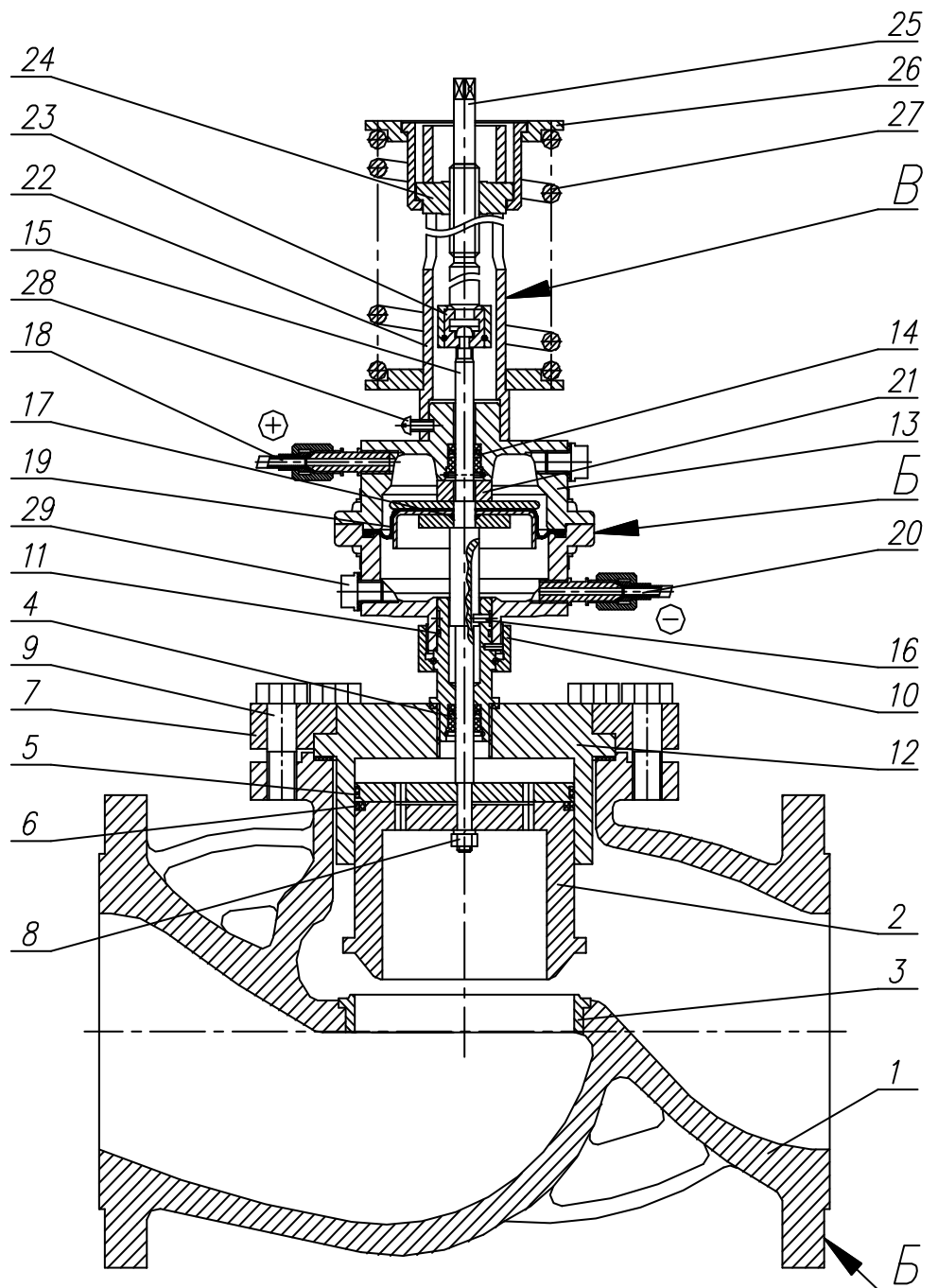
Рисунок 1. Общее устройство регулятора РП-125.
