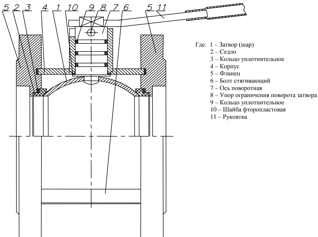
Рисунок 1. Общее устройство крана
