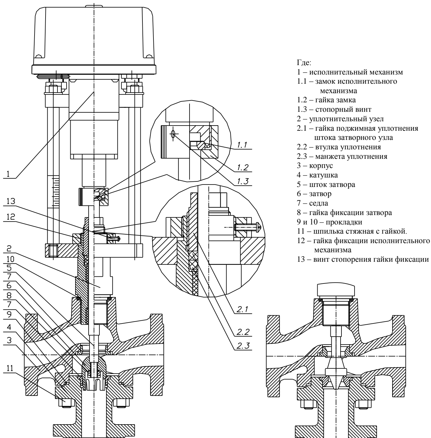
Рисунок 1. Общее устройство клапана смесительного трехходового КСТ-XX/XX.X-XX
