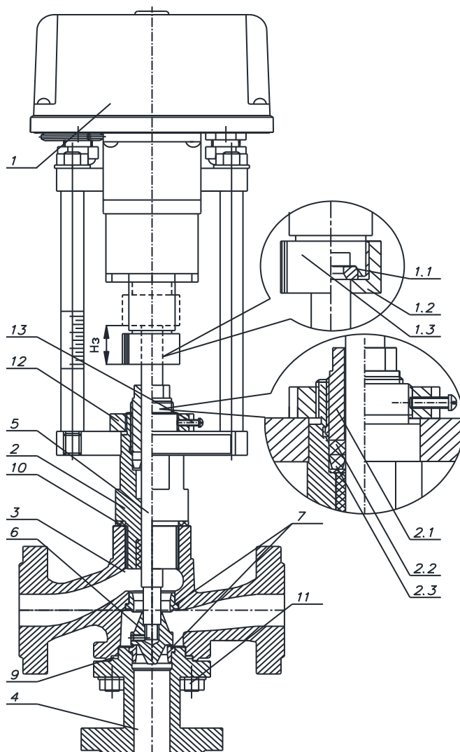
Рисунок 1. Общее устройство клапана смесительного трехходового КСТ-20/XX.B
