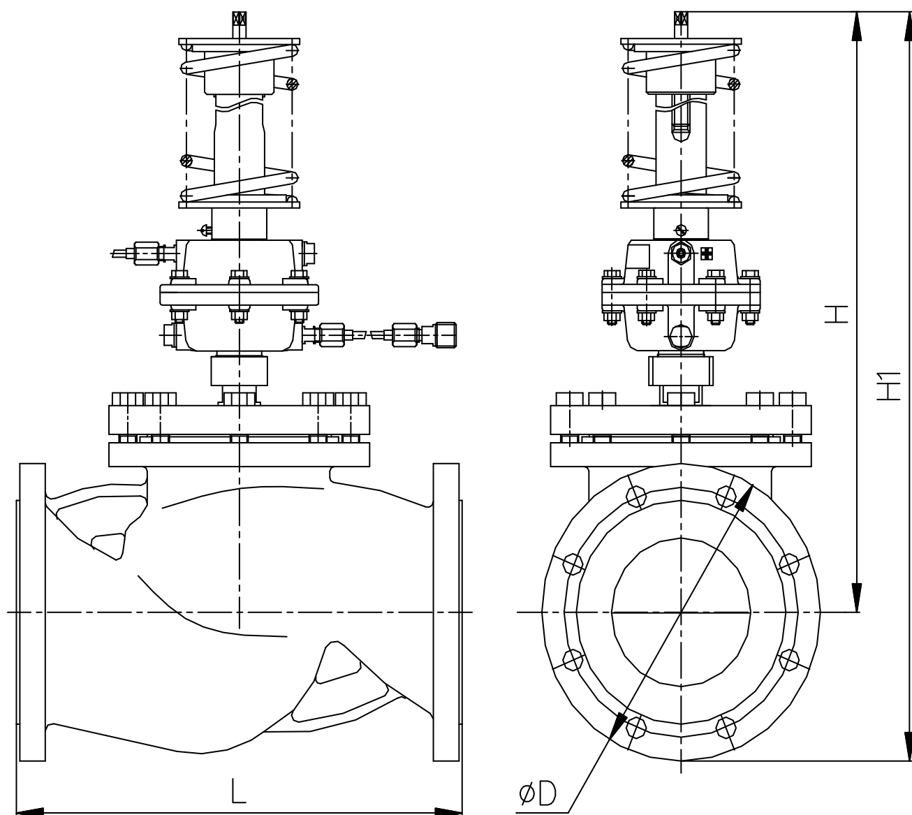
Рисунок 1. Общий вид регулятора.
