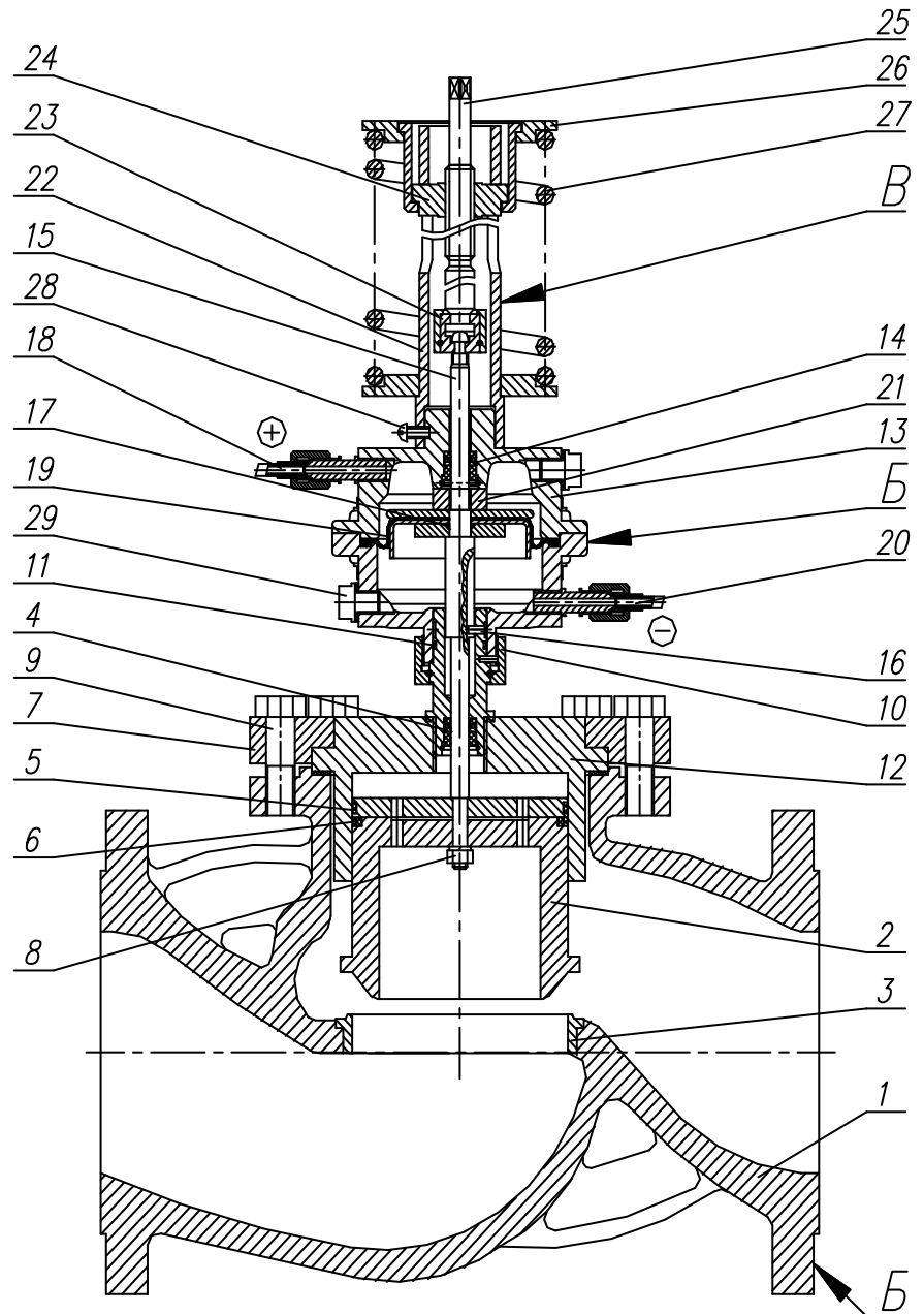
Рисунок 1. Общее устройство регулятора РД-А-125.
